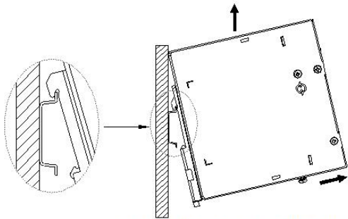
④接着第③步骤，先把产品本体底部往推， 再将其往上提，即可把产品从导轨上取出。
