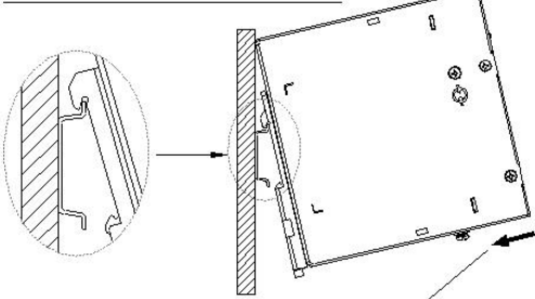
②把产品本体垂直TS35导轨方向推， 直到听到卡扣卡入导轨的声音;
