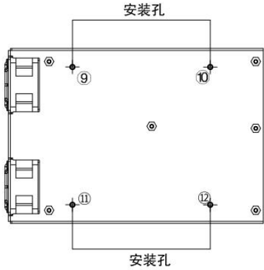
底视图
